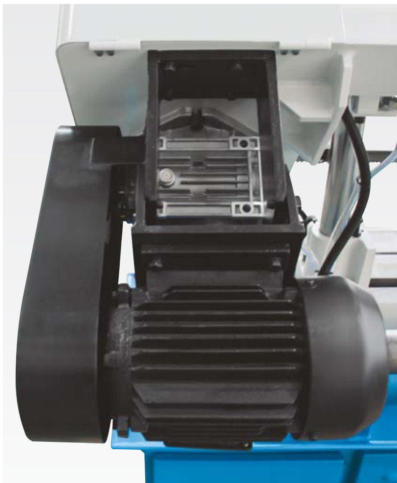
Привод с клиновидным ремнем для НВ 280 Т
